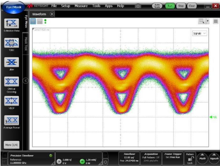
MXIQ-LN-30 | 22Gubd QPSK调制
